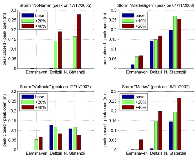
Figuur 5.4. De toename van de hoogste waterstand veroorzaakt door het sluiten van het Emssperrwerk voor Eemshaven, Delfzijl en Nieuwe Statenzijl. Elk blok representeert één van de stormsituaties. "Base" is de simulatie die het beste overeenkomt met de waarnemingen. De groene en bruine staafjes geven de simulaties waarvoor de windsnelheden met de aangegeven percentages zijn verhoogd. Overgenomen uit De Lima Rego en Dillingh (2010).
