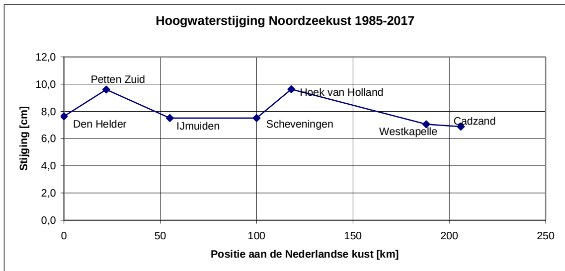
Figuur 4.1 Ruimtelijke verdeling toeslagen Hollandse en Zeeuwse Noordzeekust
