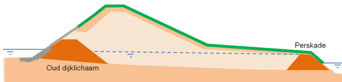
Figuur 5.1 Schematische weergave van dijkopbouw waarbij het freatisch vlak onder dagelijkse omstandigheden hoger is dan op basis van polderpeil en gemiddeld buitenpeil mag worden verwacht.
