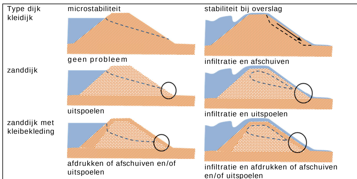
Figuur 3.1 Schematische weergave verschillen en overeenkomsten microstabiliteit en stabiliteit van de bekleding bij golfoverslag
