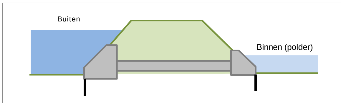
Figuur 7-1 Globale schets van doorsnede dijk met uitwateringssluis
