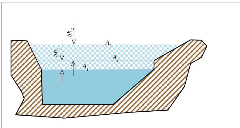
Figuur 7-2 Schematische weergave dwarsdoorsnede voor voorbeeld
