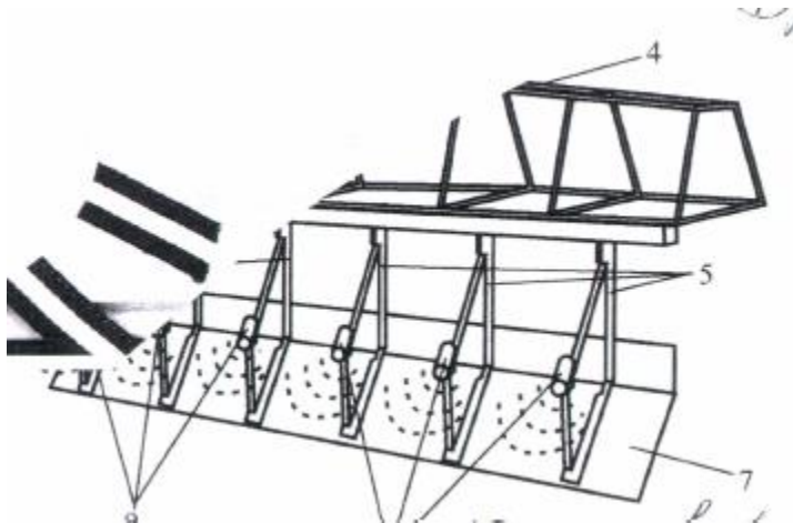
Figuur 1: Wingssprayer type Single Wing-systeem, waarbij de spuitdoppen zijn verbonden met de vleugels (Wings)
