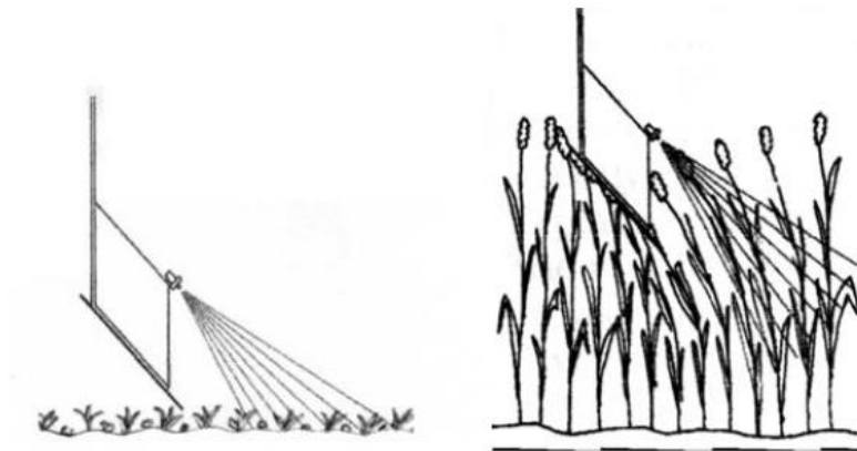
Figuur 3: Het werkingsprincipe van Wingssprayer op een jong gewas en in een vol gewas (Enfält et al. 2000)
