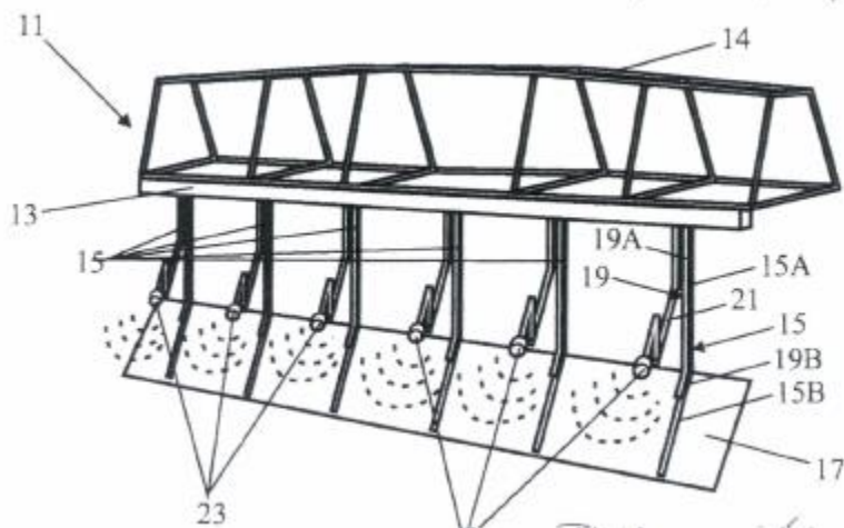
Figuur 2: Wingssprayer type Single Wing-systeem, waarbij de spuitdoppen niet zijn verbonden met de vleugels (Wings)
