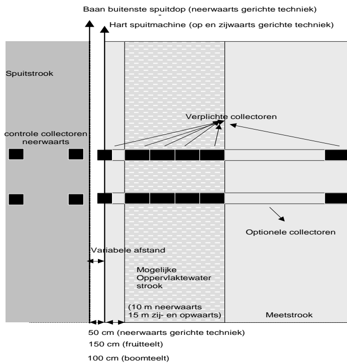
Figuur 3. Schematische weergave van de veldmetingen en de plaats van de collectoren
