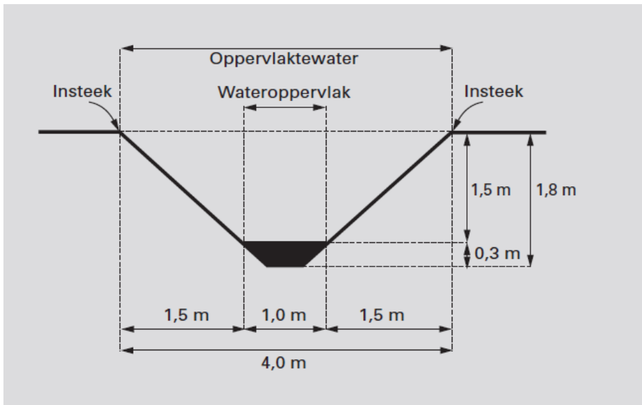
Figuur 1. Schematische weergave van standaardsgoot.
