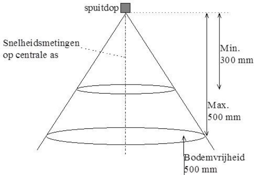
Figuur 1 Druppelgroottemetingen bij een spuitdop in een horizontaal vlak op 30 tot 50 cm onder de spuitdop. Het meetvlak moet zich ten minste 50 cm boven het grondoppervlak bevinden.
