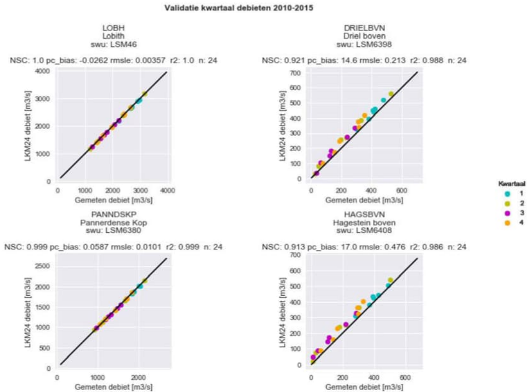
Figuur B11.3 Meetpunten langs de Rijn, Nederrijn en Lek: berekend debiet (y-as) versus gemeten debiet (x-as).
