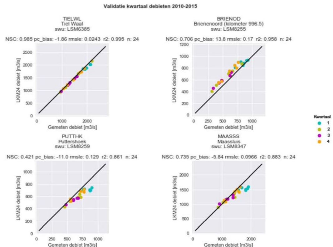
Figuur B11.4 Meetpunten langs de Waal, Oude en Nieuwe Maas: berekend debiet (y-as) versus gemeten debiet (x-as).
