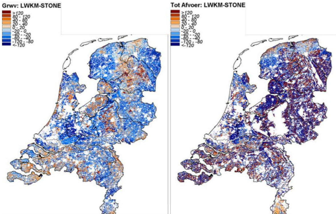
Figuur 6.2 Verskil tussen door LWKM en STONE berekende grondwatervoeding (links) en waterafvoer uit de bodem (rechts) in mm/jr. Bij getallen groter dan 0 is de LWKM-waarde groter dan de STONE-waarde en bij getallen kleiner dan 0 is de LWKM-waarde kleiner dan de STONE-waarde.
