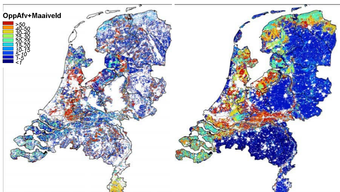
Figuur B6.10 Oppervlakkige afstroming + maaiveld drainage (mm/jr) in de periode 1981-2010 in LHM (links) en in STONE (rechts).
