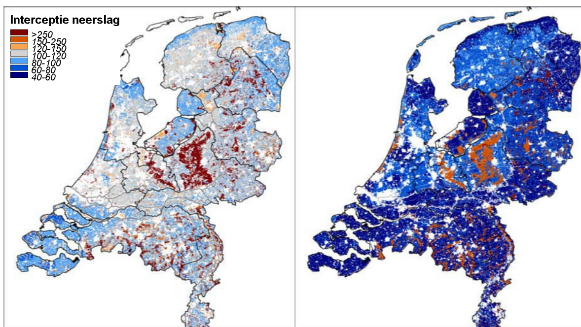
Figuur B6.6 Interceptie (mm/jr) in de periode 1981-2010 in LHM (links) en in STONE (rechts).
