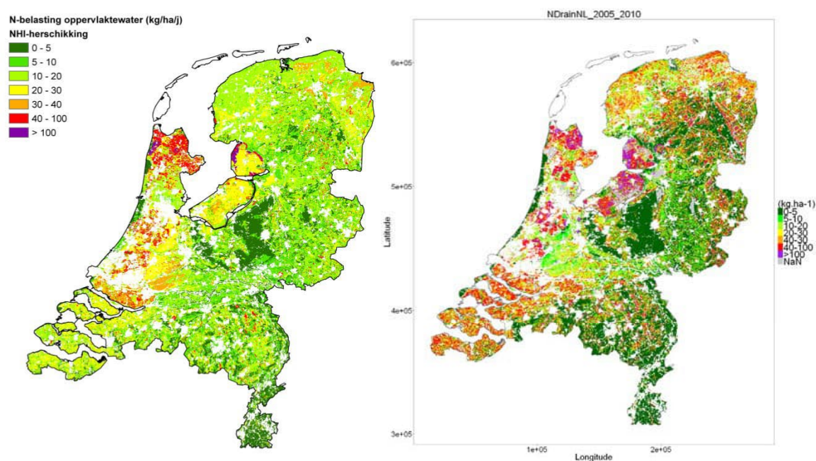
Figuur 4.8 Belasting van het oppervlaktewater met totaal-stikstof voor de periode 2005-2010 berekend met LHM3.3 en LWKM met geactualiseerde bodemparameters, maar zonder aangepaste kwelconcentratie op de onderrand en zonder nieuwe initialisatie.
