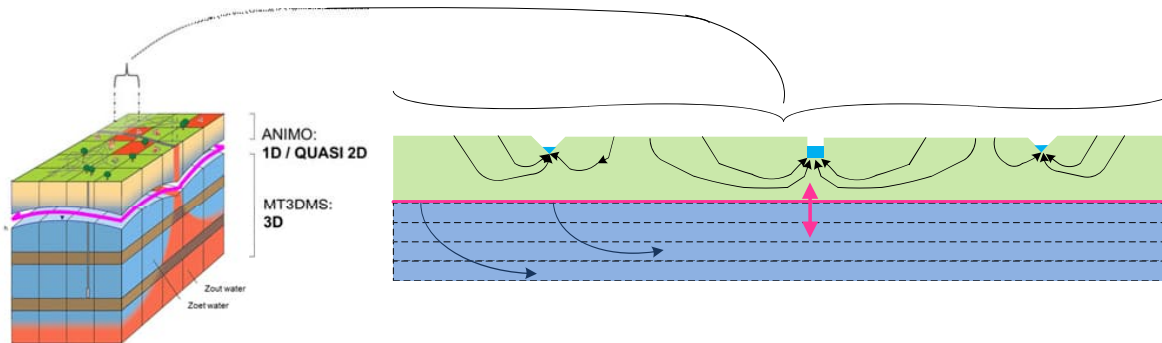
Figuur 2.4 Het koppelingsconcept tussen ANIMO en MT3DMS. Links geeft de koppeling van het grondwatermodel in rekeneenheden weer, rechts op één enkele modelkolom.
