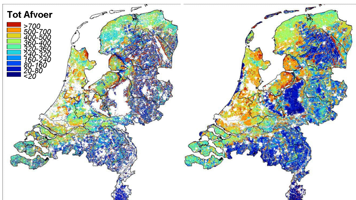
Figuur B6.16 Totale afvoer uit de bodem (mm/jr) in de periode 1981-2010 in LHM (links) en in STONE (rechts).
