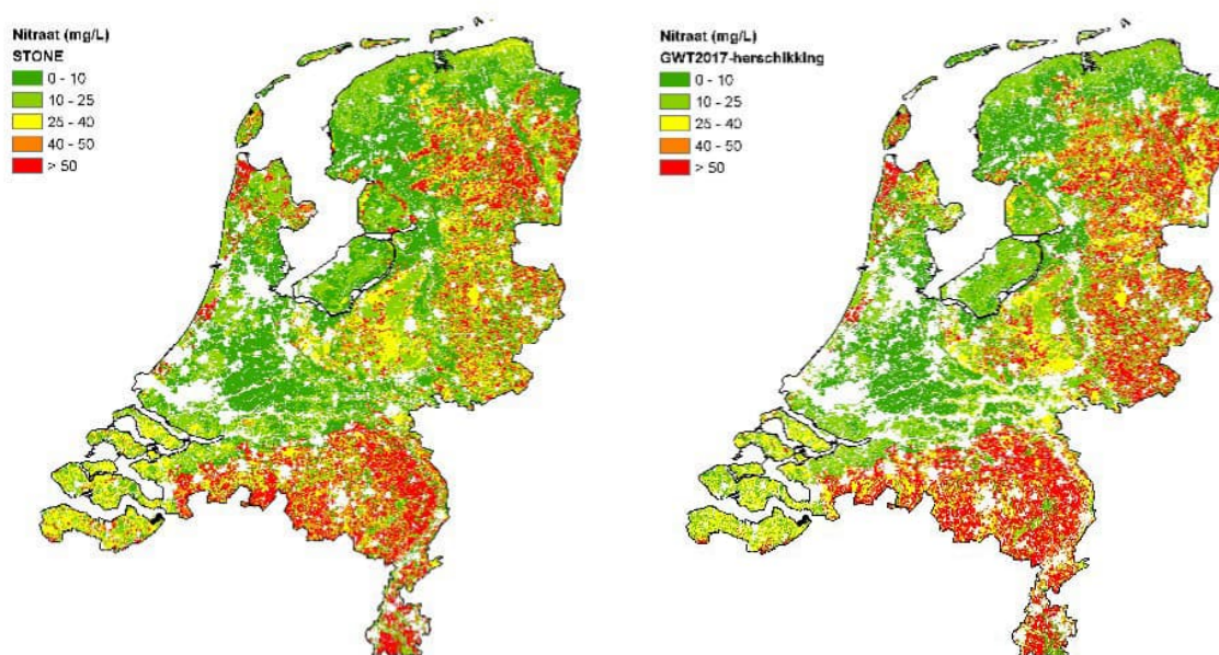
Figuur 4.1 Nitraatconcentraties in het bovenste grondwater voor de periode 2005-2010 berekend met STONE (links) en voor STONE geprojecteerd op de geactualiseerde Gt-kaart, buisdrainage en landgebruik (rechts).
