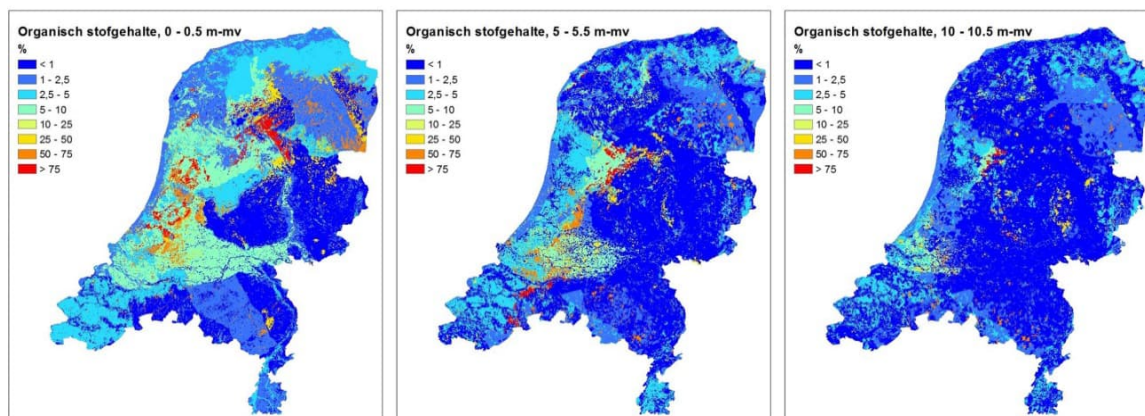
Figuur 3.5 Organischestofgehaltes in het geochemisch voxelmodel op drie diepteniveaus.
