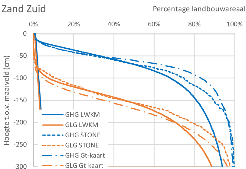
Figuur B6.23 Vergelijking van GHG en GLG-waarden van landbouwgronden in LHM, in STONE en van de landbouwpercelen in BRP2016 waarvoor de grondwatertrappenkaart (rapport 2797) een waarde heeft, voor de drie zandgebieden in het LMM.
