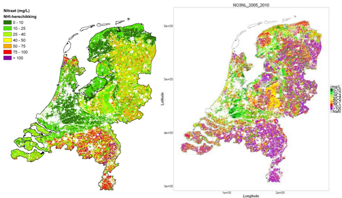
Figuur 4.7 Nitraatconcentraties in het bovenste grondwater voor de periode 2005-2010 berekend met LHM3.3 en LWKM met geactualiseerde bodemparameters, maar zonder aangepaste kwelconcentratie op de onderrand en zonder nieuwe initialisatie.
