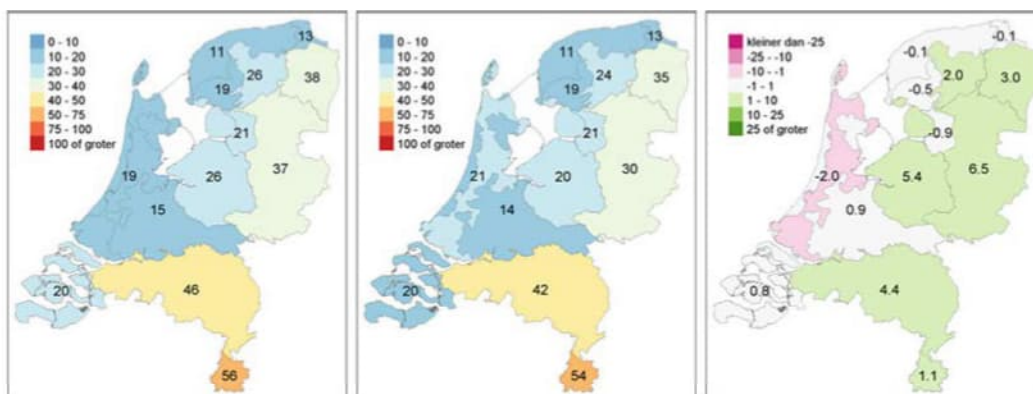
Figuur 7.6 Nitraatconcentraties (mg/L) onder landbouw, gemiddeld per grondwaterlichaam in 2027, berekend met de volledige set aan Landbouw-rekenenheden (links) en bij vervanging van waarden van rekenenheden met een extreme hydrologie door het gebiedsgemiddelde (midden). Het effect hiervan is rechts weergegeven.
