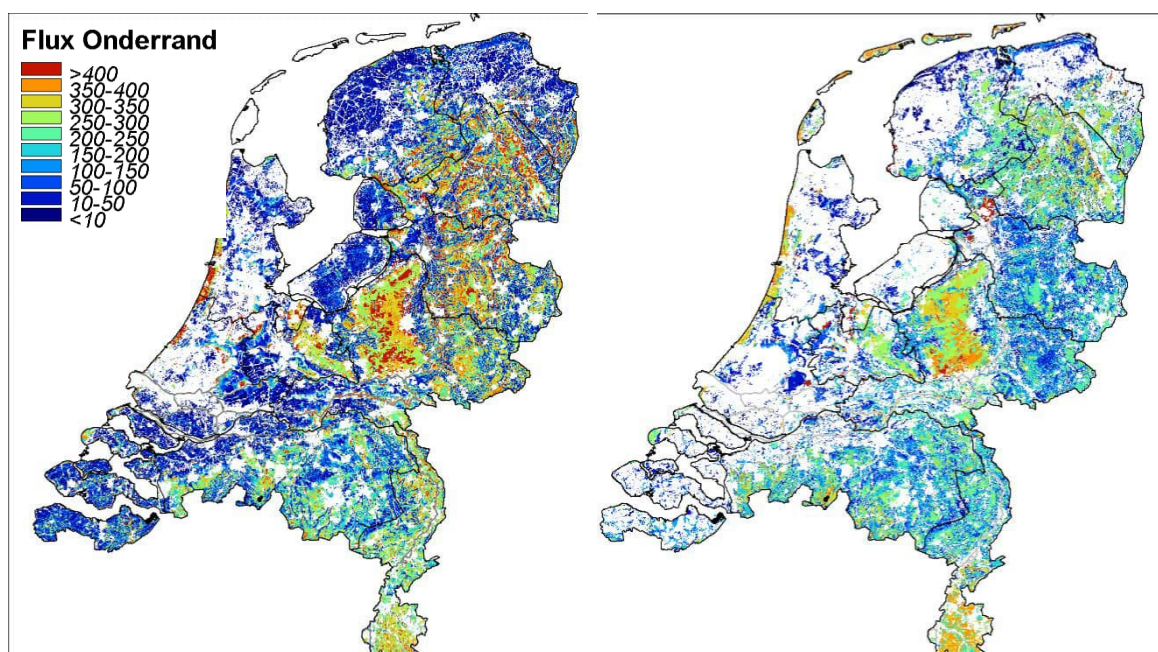
Figuur B6.18 Onderrand flux neerwaarts (mm/jr) in de periode 1981-2010 in LHM (links) en in STONE (rechts).
