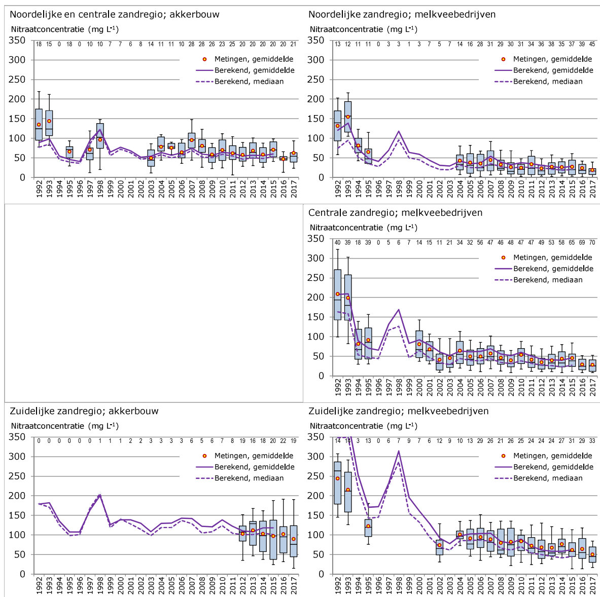
Figuur 6.12 Vergelijking van berekende gemiddelde en mediaanwaarden van de nitraatconcentratie in de eerste meter van het grondwater op landbouwbedrijven in de zandregio's met metingen in het LMM. De box-whisker diagrammen geven de 10-, 25-, 50-, 75- en 90-percentielwaarden van de metingen weer.
