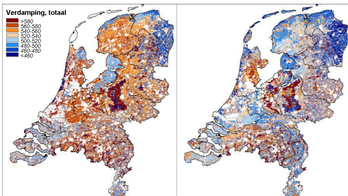
Figuur B6.4 Verdamping totaal (mm/jr) in de periode 1981-2010 in LHM (links) en in STONE (rechts).
