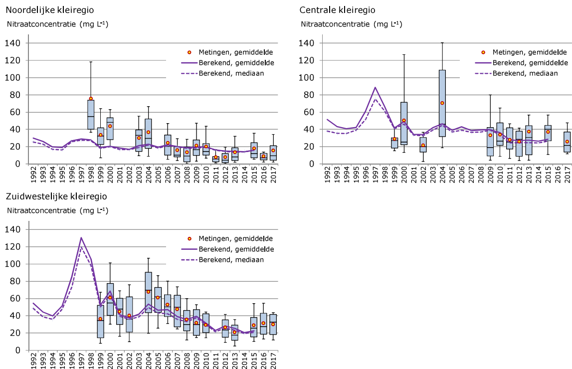
Figuur 6.20 Vergelijking van berekende gemiddelde en de mediaanwaarde van de nitraatconcentratie in drainagewater in de kleigebieden met metingen in het LMM. De box-whiskerdiagrammen geven de 10-, 25-, 50-, 75- en 90-percentielwaarden van de metingen weer.
