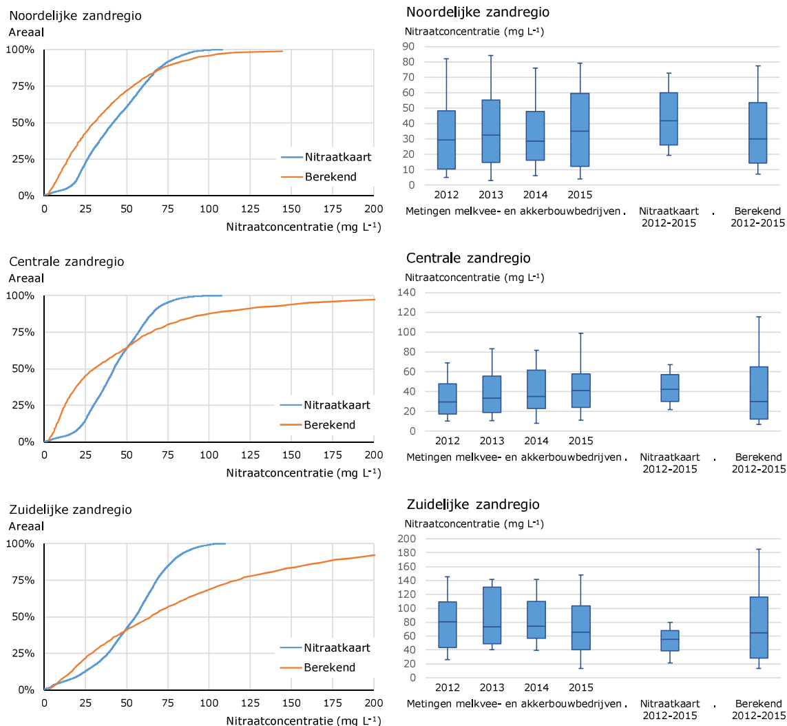
Figuur 6.10 Cumulatieve frequentieverdeling voor LWKM en de Nitratkaart (RIVM 2018) voor drie zandregio's.
