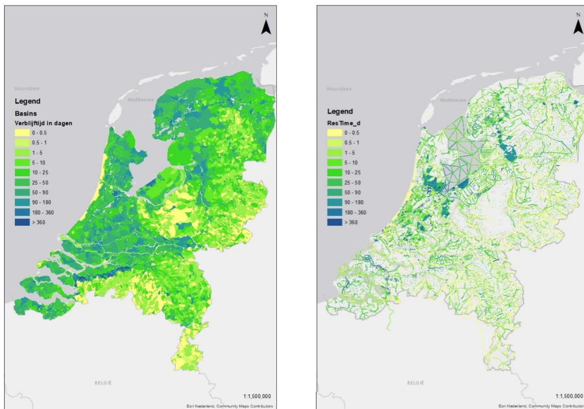
Figuur B12.1 Verblijftijden in dagen voor de basin knooppunten (links) en SWU's (rechts) van de LKM 2.4-schematisering, zoals berekend voor het tweede kwartaal van 2015.
