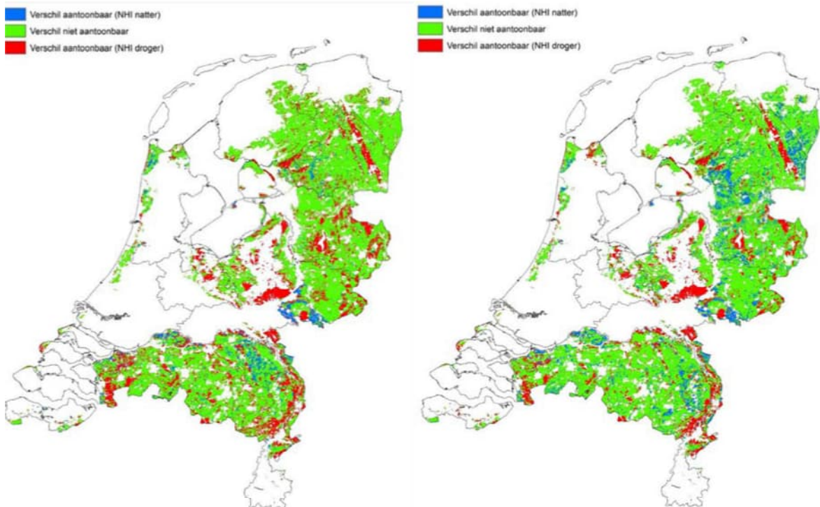
Figuur 5.2 Zones waar in het pleistocene deel van Nederland de met LHM 3.5 berekende GHG's (links) en GLG's (rechts) aantoonbaar dieper of ondieper zijn dan de Gd-kaart.
